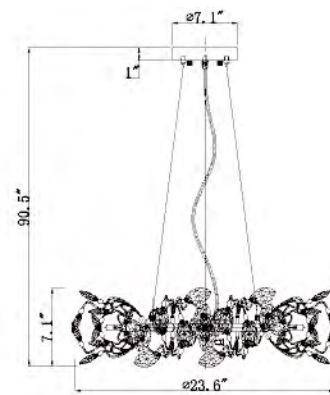
ZL22W12MN E12×6 Max40W
