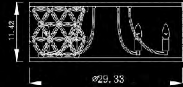
ZL35F29CH E12×12 Max40W
